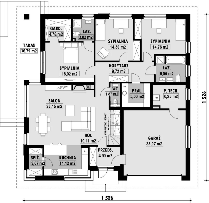
RZUT PARTERU
