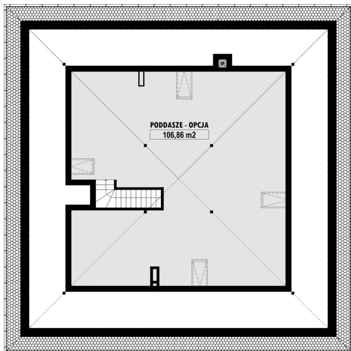
E-262 PODDASZE E-262 PODDASZE - OPCJA
