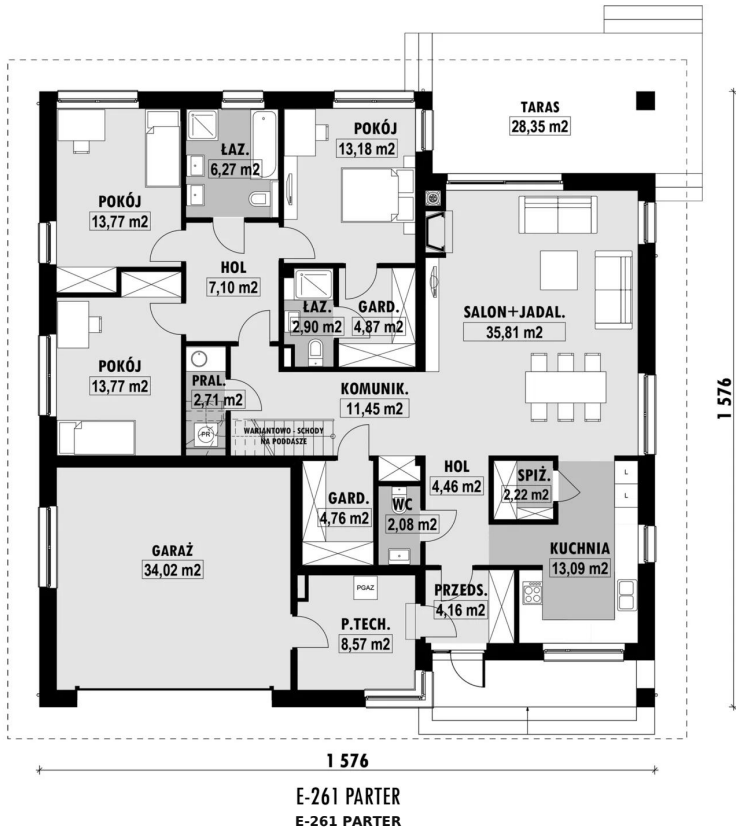
RZUT PARTERU
