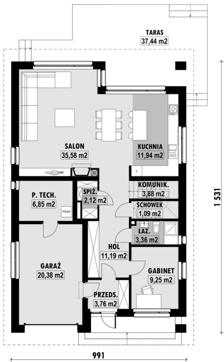
RZUT PARTERU
