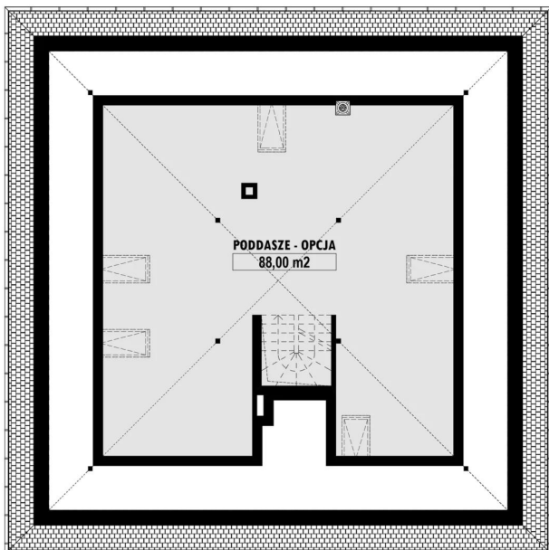
E-244a PODDASZE E-244a PODDASZE - OPCJA
