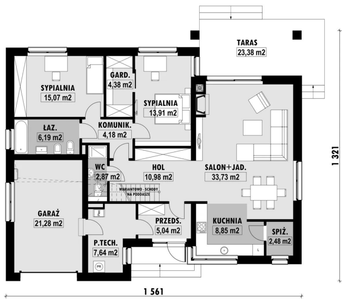
RZUT PARTERU
