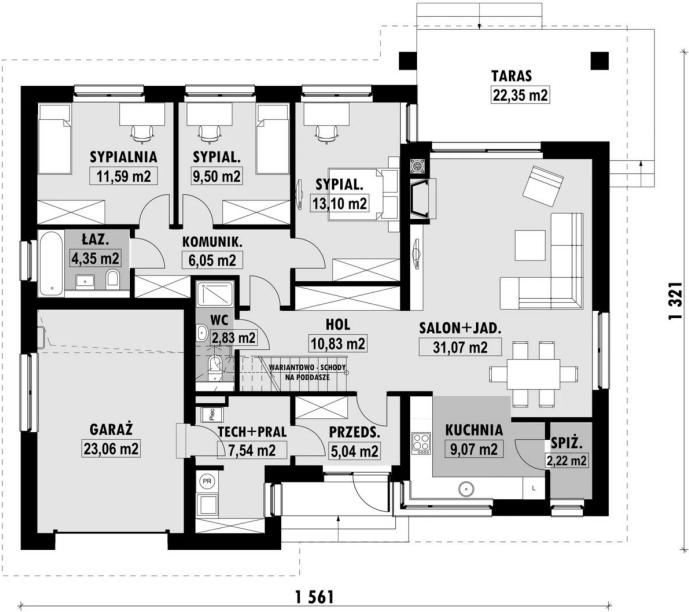
RZUT PATERU
