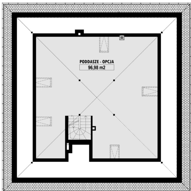
E-240 PODDASZE E-240 PODDASZE - OPCJA
