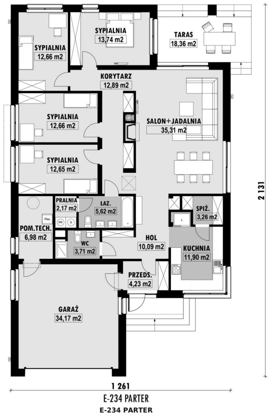
RZUT PARTERU
