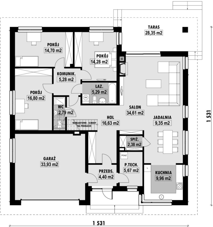
E-232 PARTER E-232 PARTER
