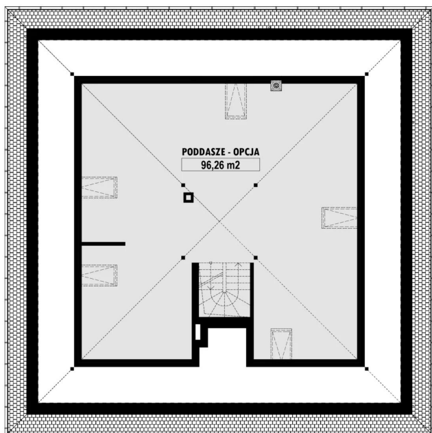
E-230 PODDASZE E-230 PODDASZE - OPCJA
