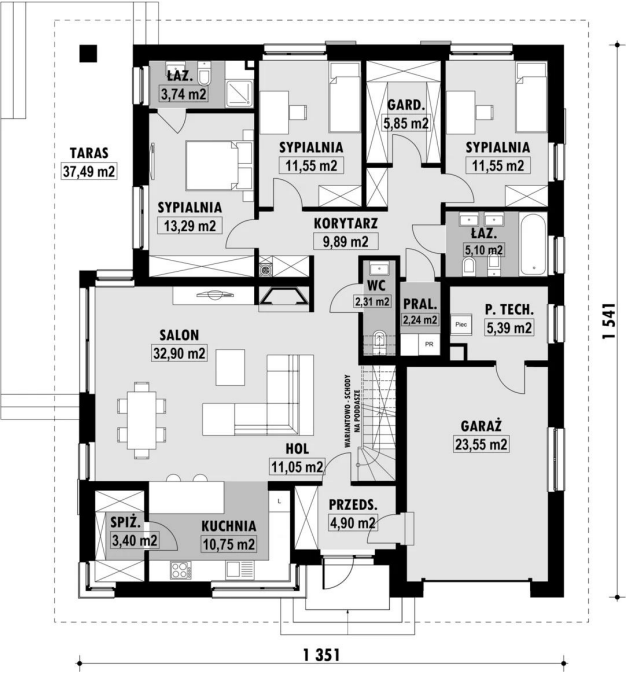
RZUT PARTERU
