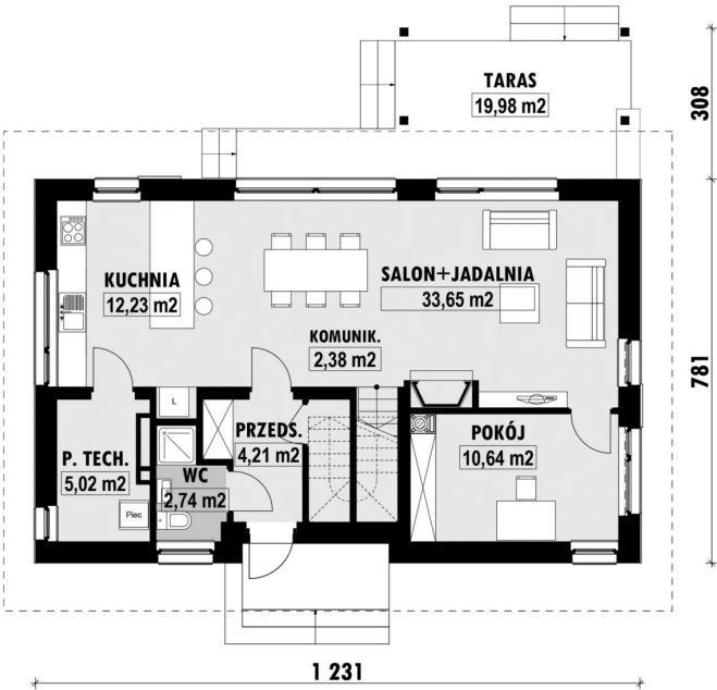
RZUT PARTERU
