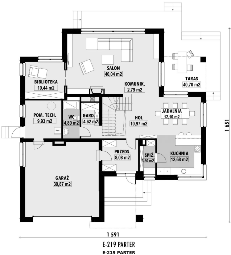
RZUT PARTERU
