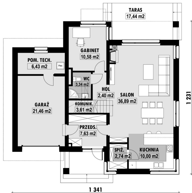
✕ RZUT PARTERU
