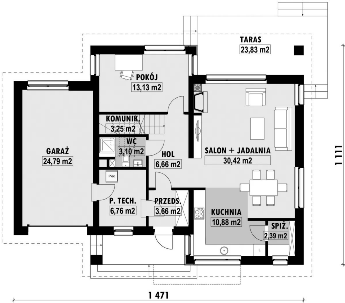
RZUT PARTERU
