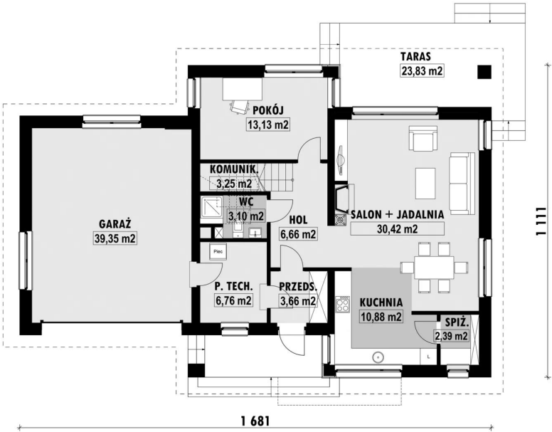
RZUT PARTERU
