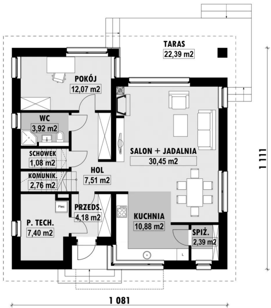
RZUT PARTERU
