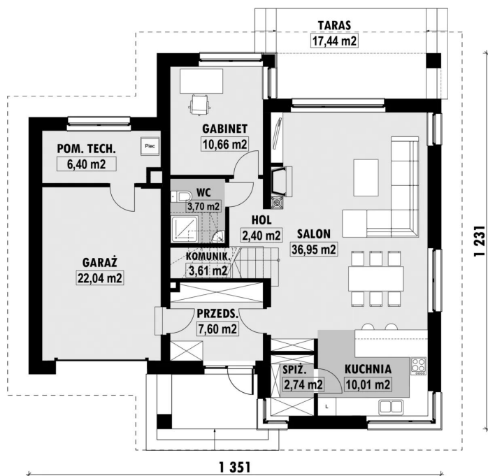
✕ RZUT PARTERU
