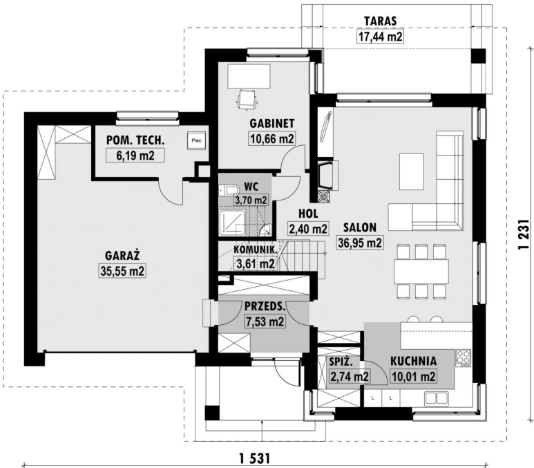
RZUT PARTERU
