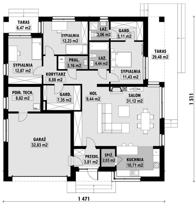
RZUT PARTERU
