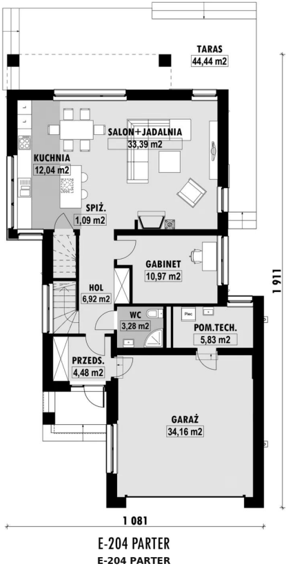
RZUT PARTERU
