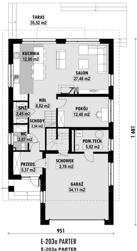
RZUT PARTERU
