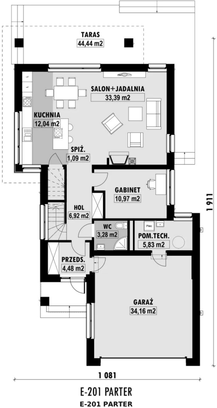
RZUT PARTERU
