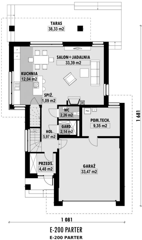
RZUT PARTERU
