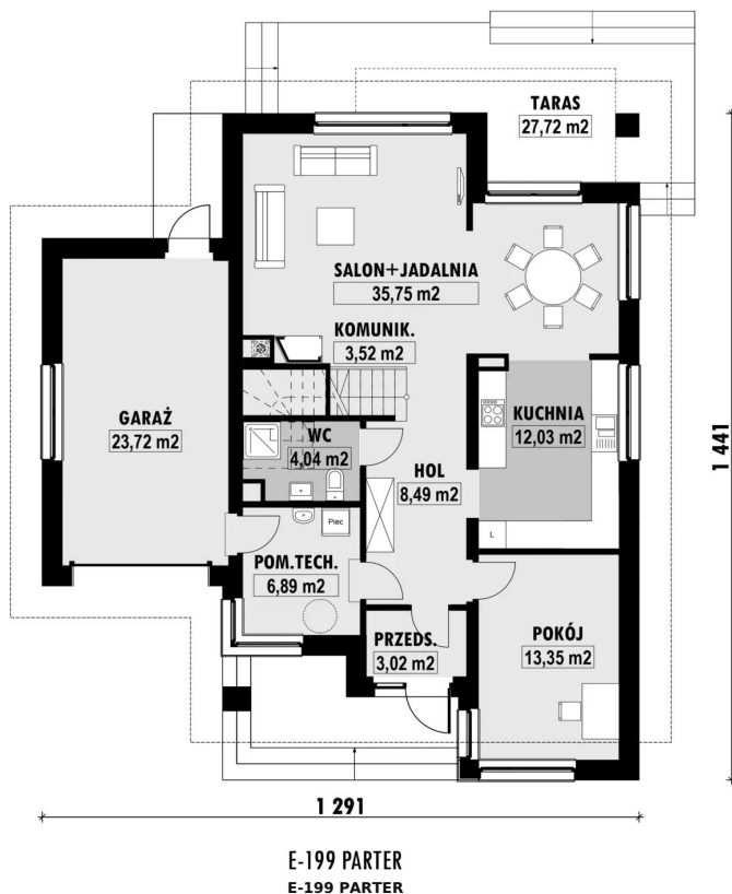
RZUT PARTERU
