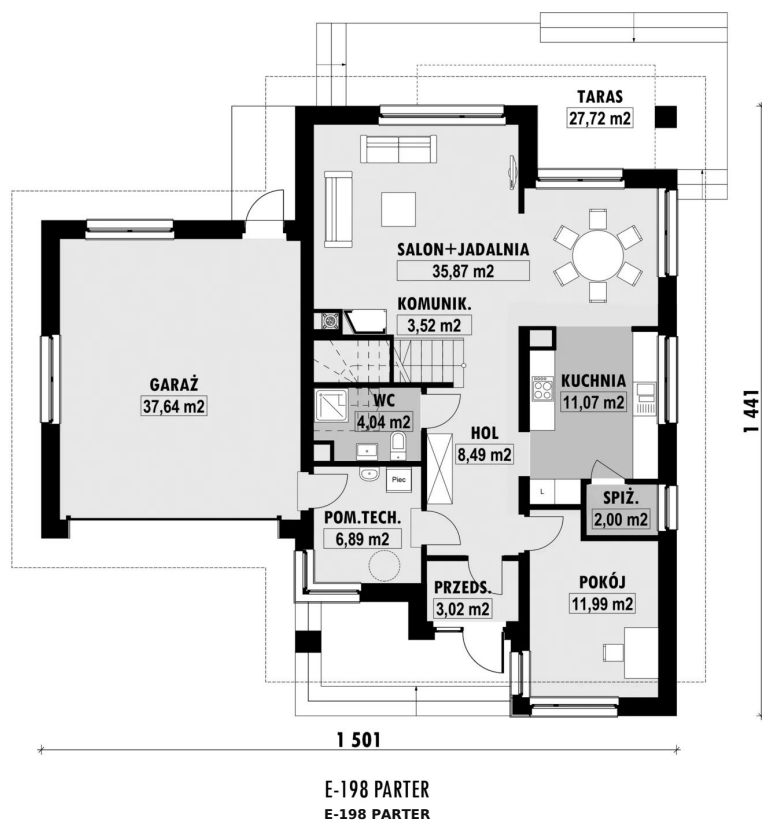
RZUT PARTERU
