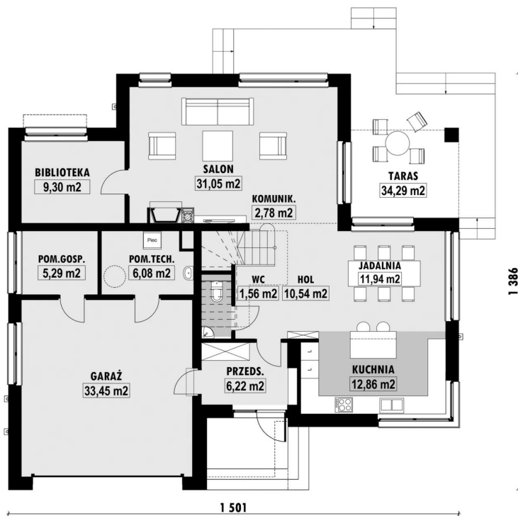
E-187 PARTER E-187 PARTER
