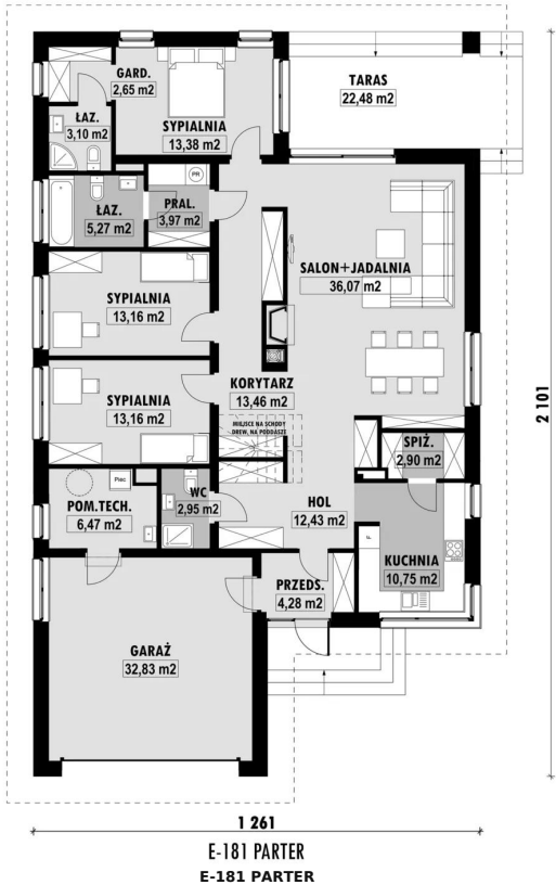
RZUT PARTERU
