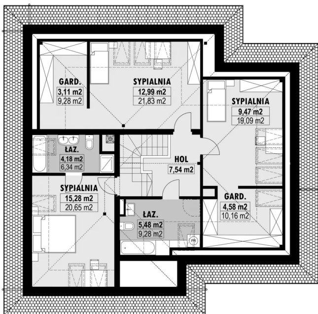
E-168 PODDASZE E-168 PODDASZE - OPCJA
