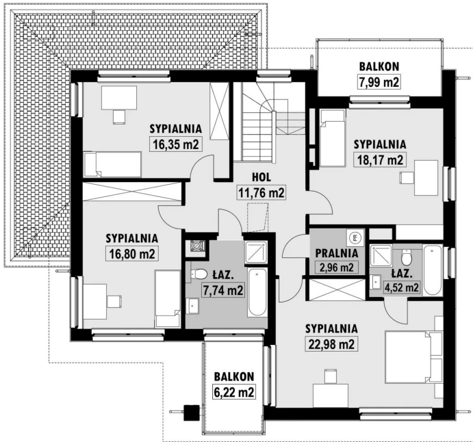
E-166 PIĘTRO E-166 PIĘTRO
