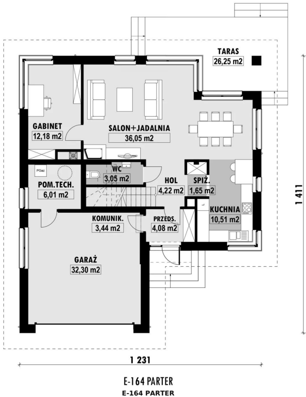
RZUT PARTERU
