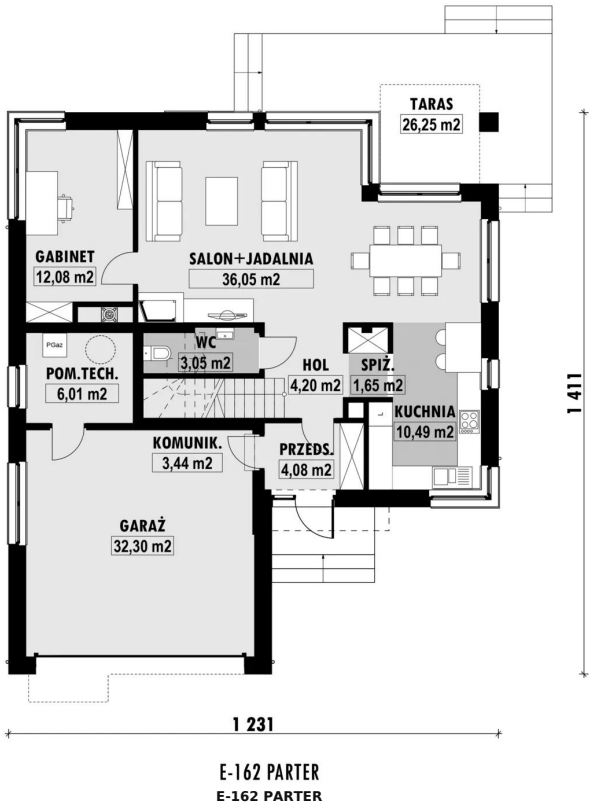
RZUT PARTERU
