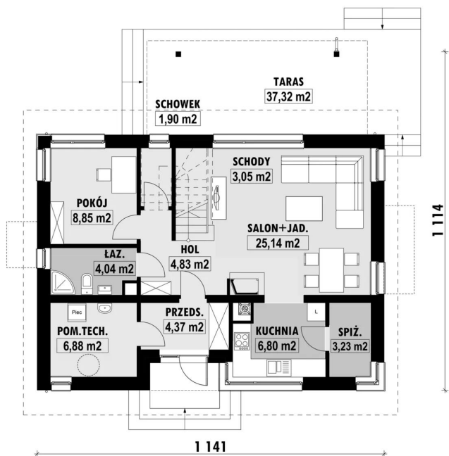
RZUT PARTERU
