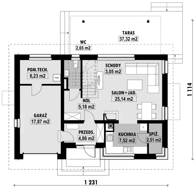
RZUT PARTERU
