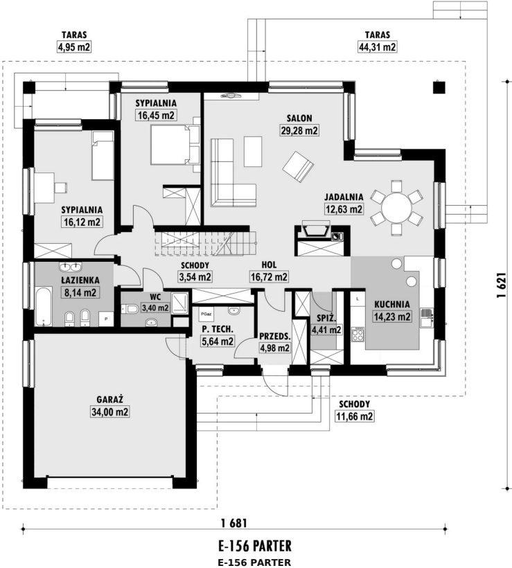
RZUT PARTERU
