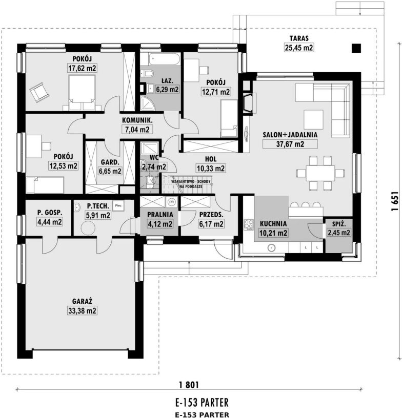
RZUT PARTERU
