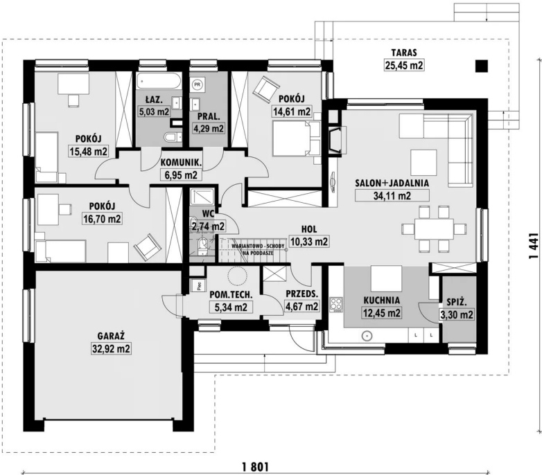
RZUT PARTERU
