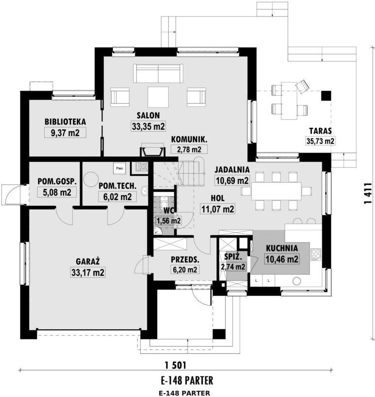
RZUT PARTERU
