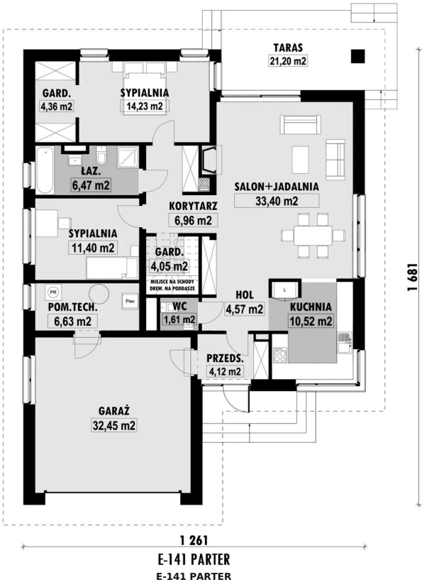
RZUT PARTERU
