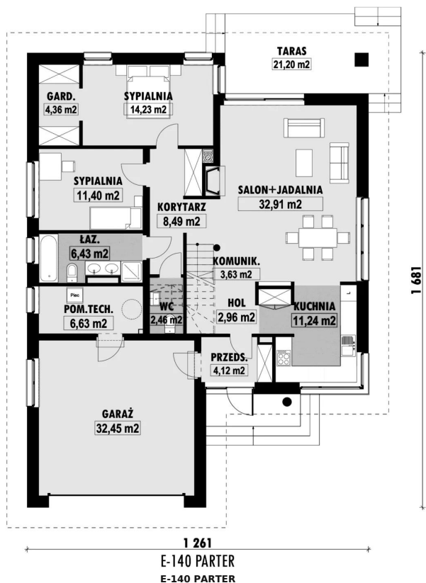
✕ RZUT PARTERU
