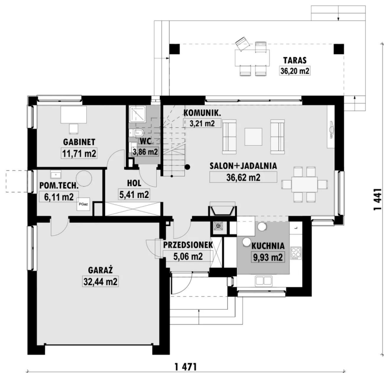
RZUT PARTERU
