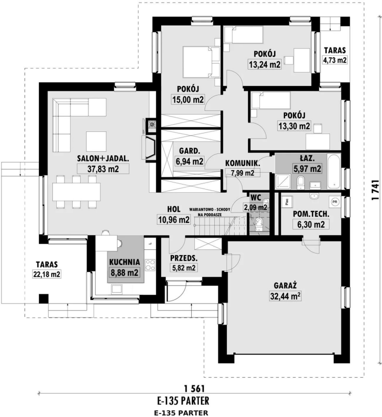
RZUT PARTERU
