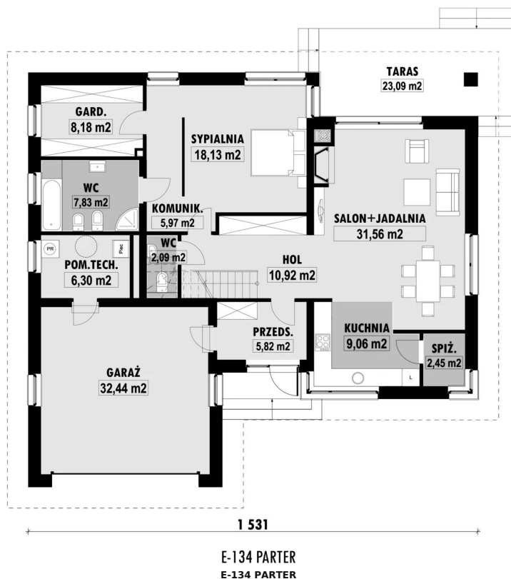
✕ RZUT PARTERU
