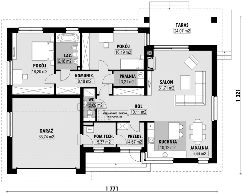
RZUT PARTERU
