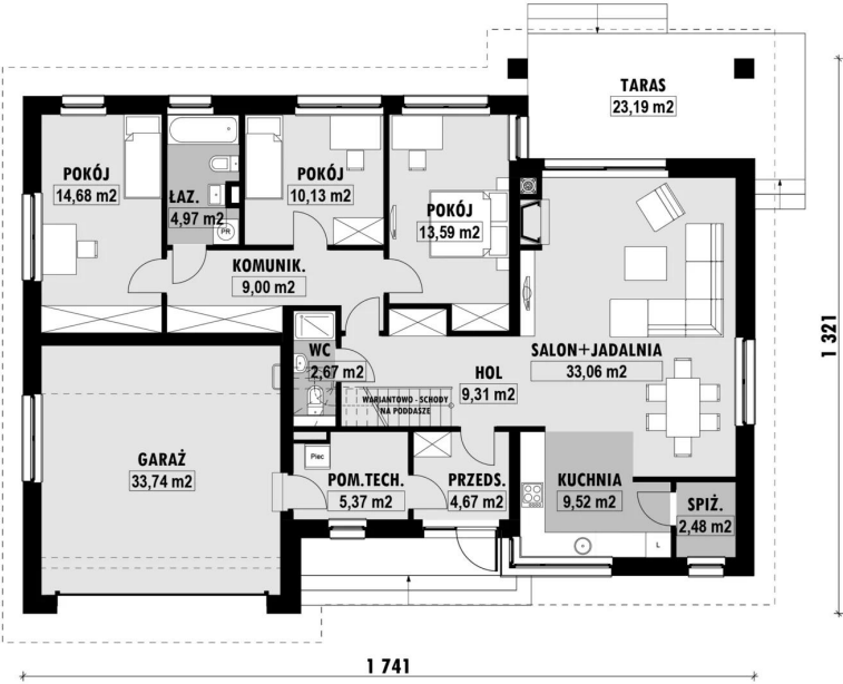
RZUT PARTERU
