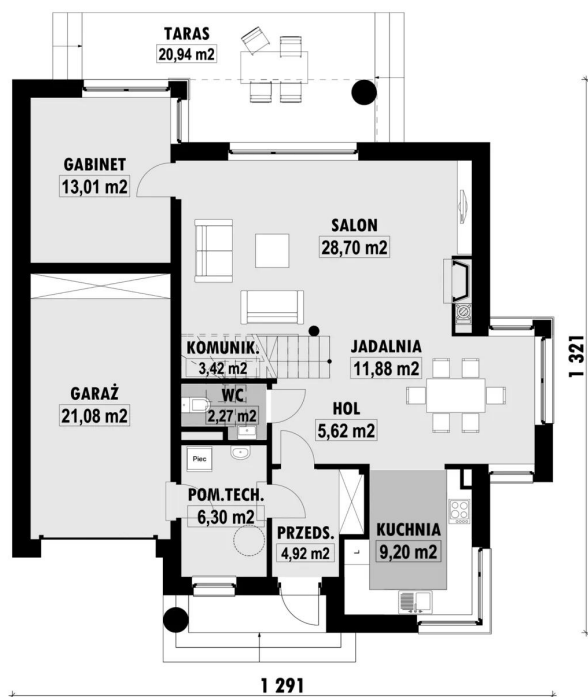
RZUT PARTERU
