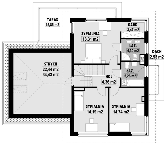
E-124 PIĘTRO E-124 PIĘTRO
