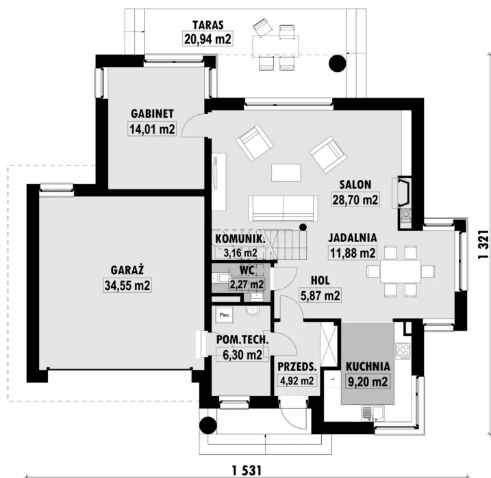
RZUT PARTERU
