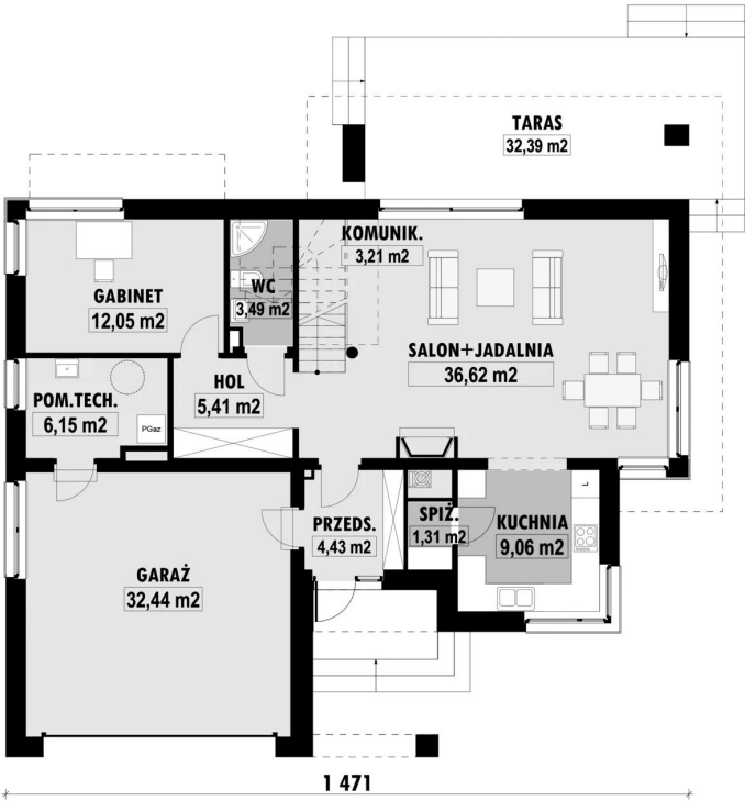
RZUT PARTERU
