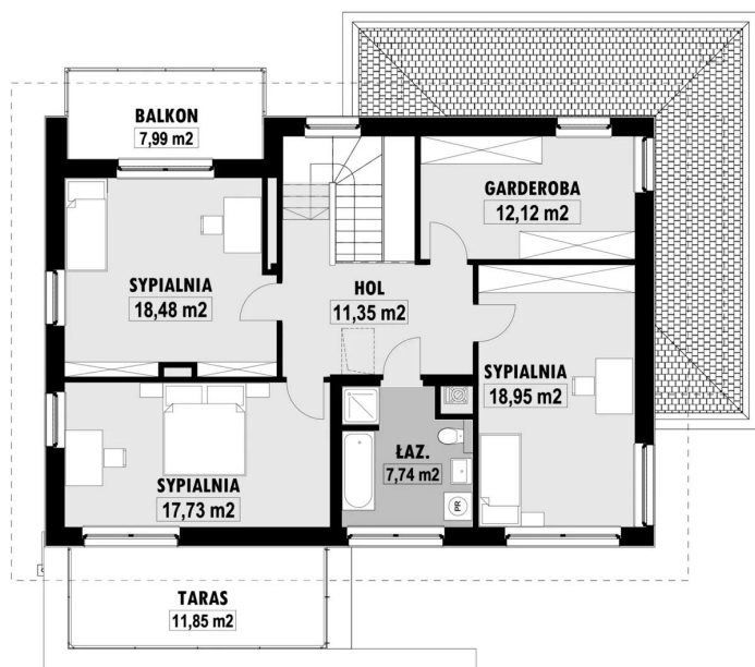
E-122 PIĘTRO E-122 PIĘTRO
