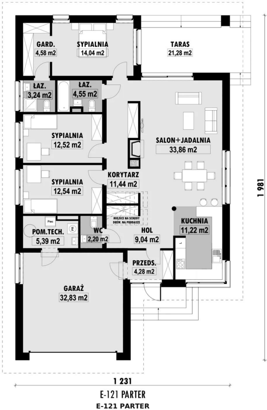
RZUT PARTERU
